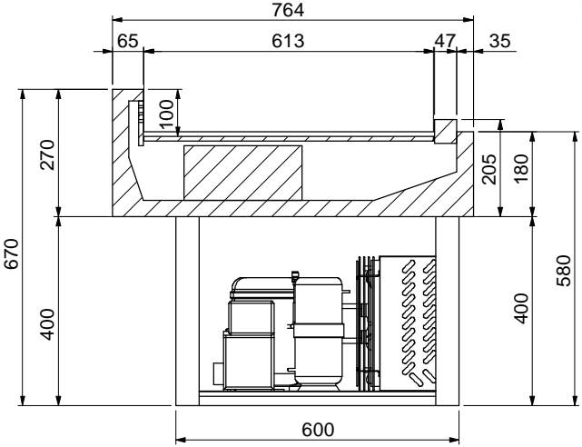
SEZIONE A-A
